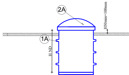
NADSTAWKI NIEPRZEJEZDNE
