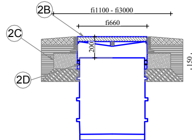
NADSTAWKI PRZEJEZDNE
