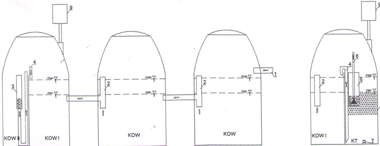
PRZEKRÓJ A-A
